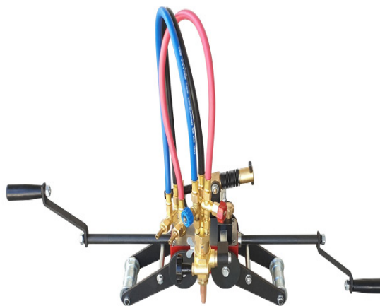
Резка труб
